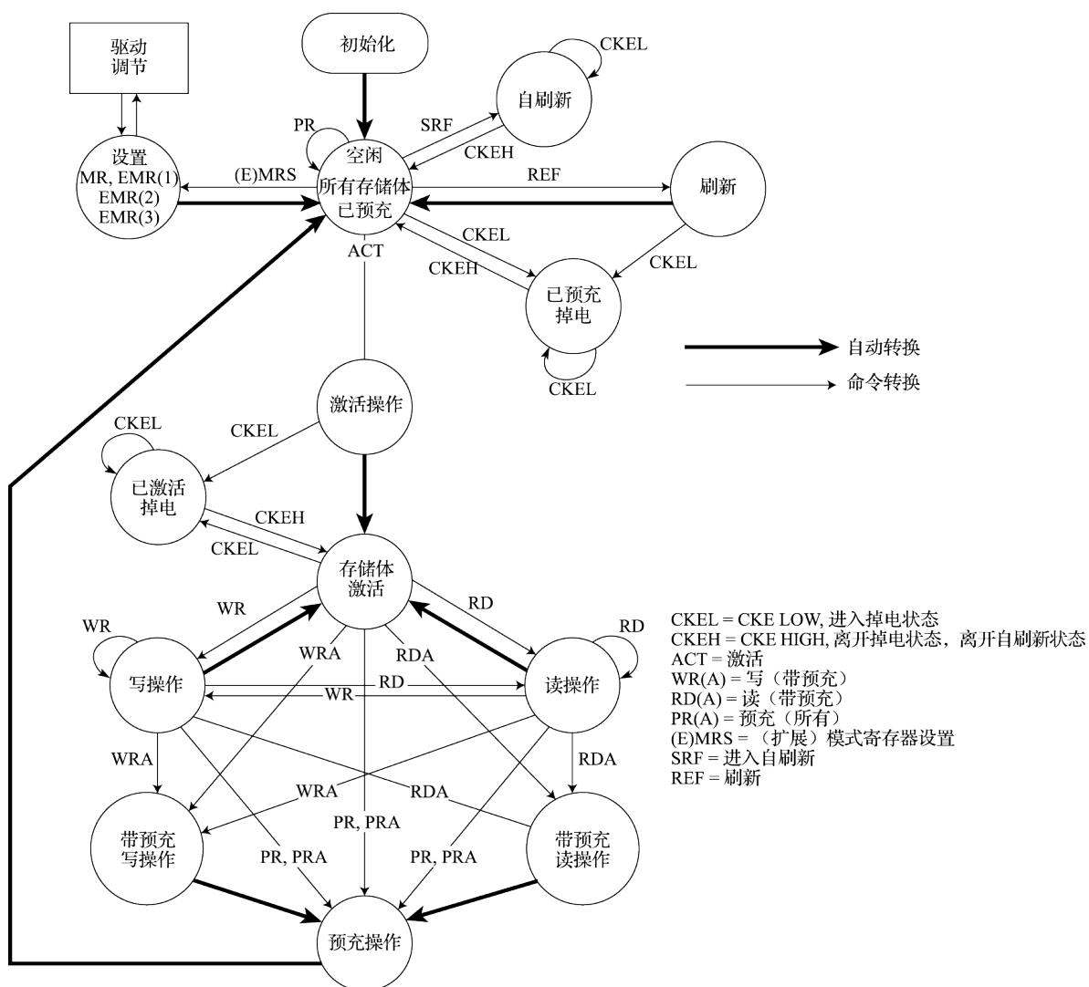
图 6.12: DDR2 内存各状态转换图
