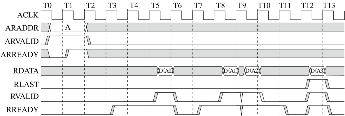
图 6.5: 突发读事务
