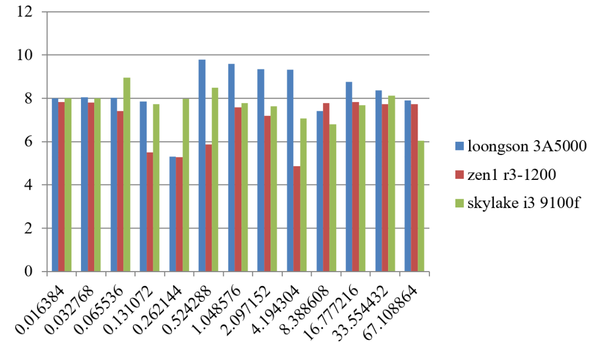
图 12.5: 访存操作的并发性
