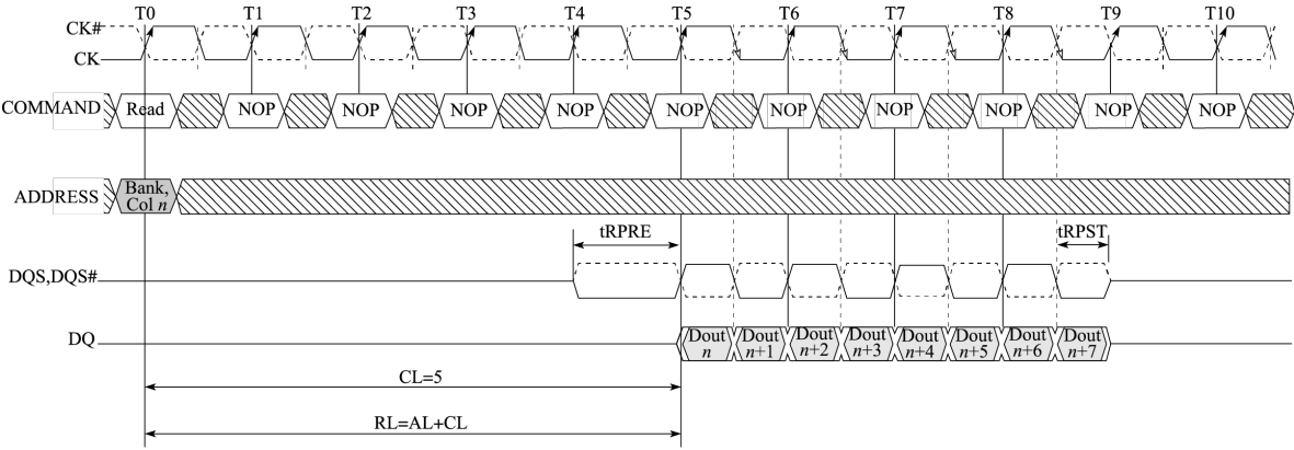
图 6.13: DDR3 SDRAM 读时序
