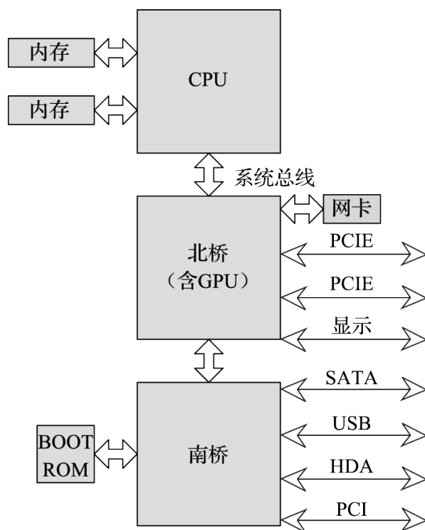
图 5.8: CPU-弱北桥-南桥结构
