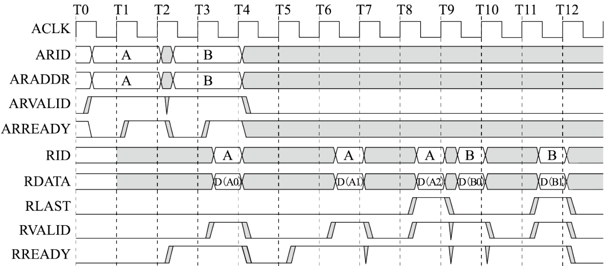
图 6.6: 重叠的读事务
