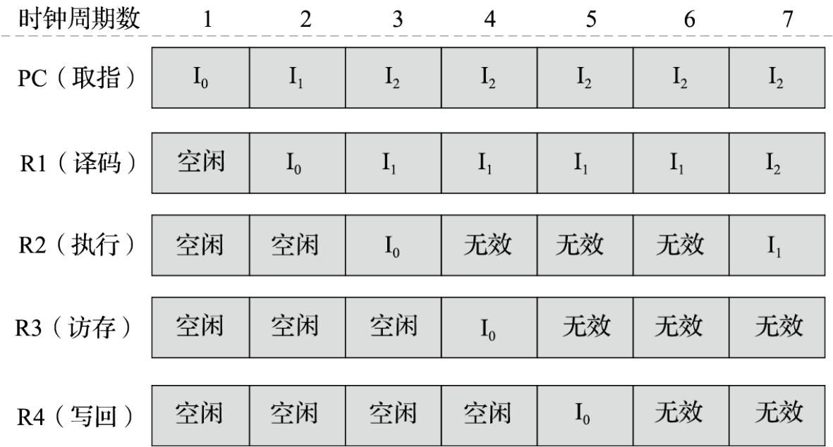
图 9.11: 有阻塞的处理器部件时空图
