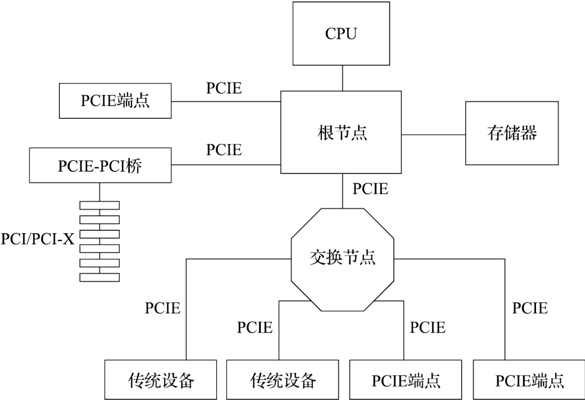
图 6.25: PCIE 接口连接示意图
