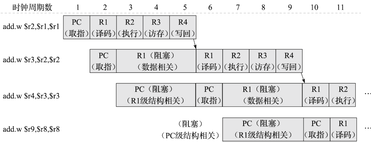
图 9.10: 用阻塞解决数据相关的流水线时空图
