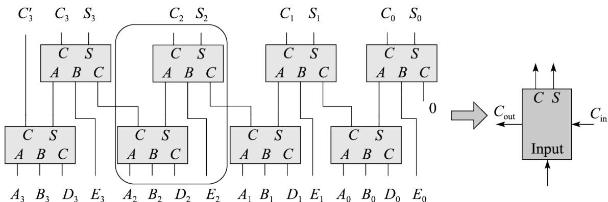
图 8.37: 使用全加器实现 4 个 4 位数相加
