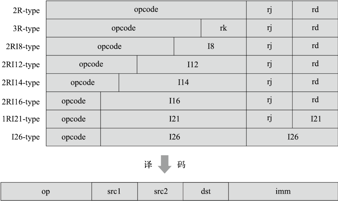
图 9.2: 译码功能示意
