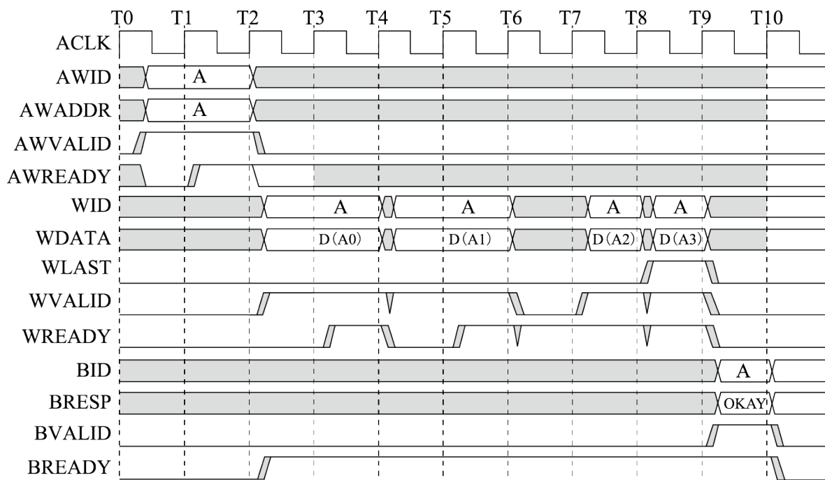
图 6.7: 写事务
