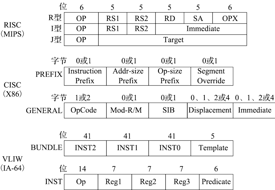
图 2.2: RISC、CISC、VLIW 指令编码特点
