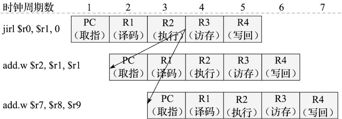
图 9.14: 控制相关示意图
