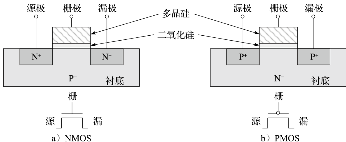
图 8.3: MOS 晶体管组成结构示意图
