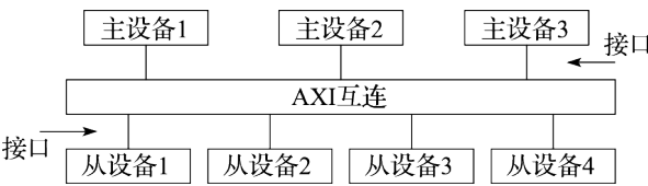
图 6.4: AXI 设备的接口和互连
