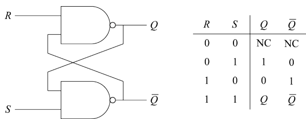
图 8.8: RS 锁存器
