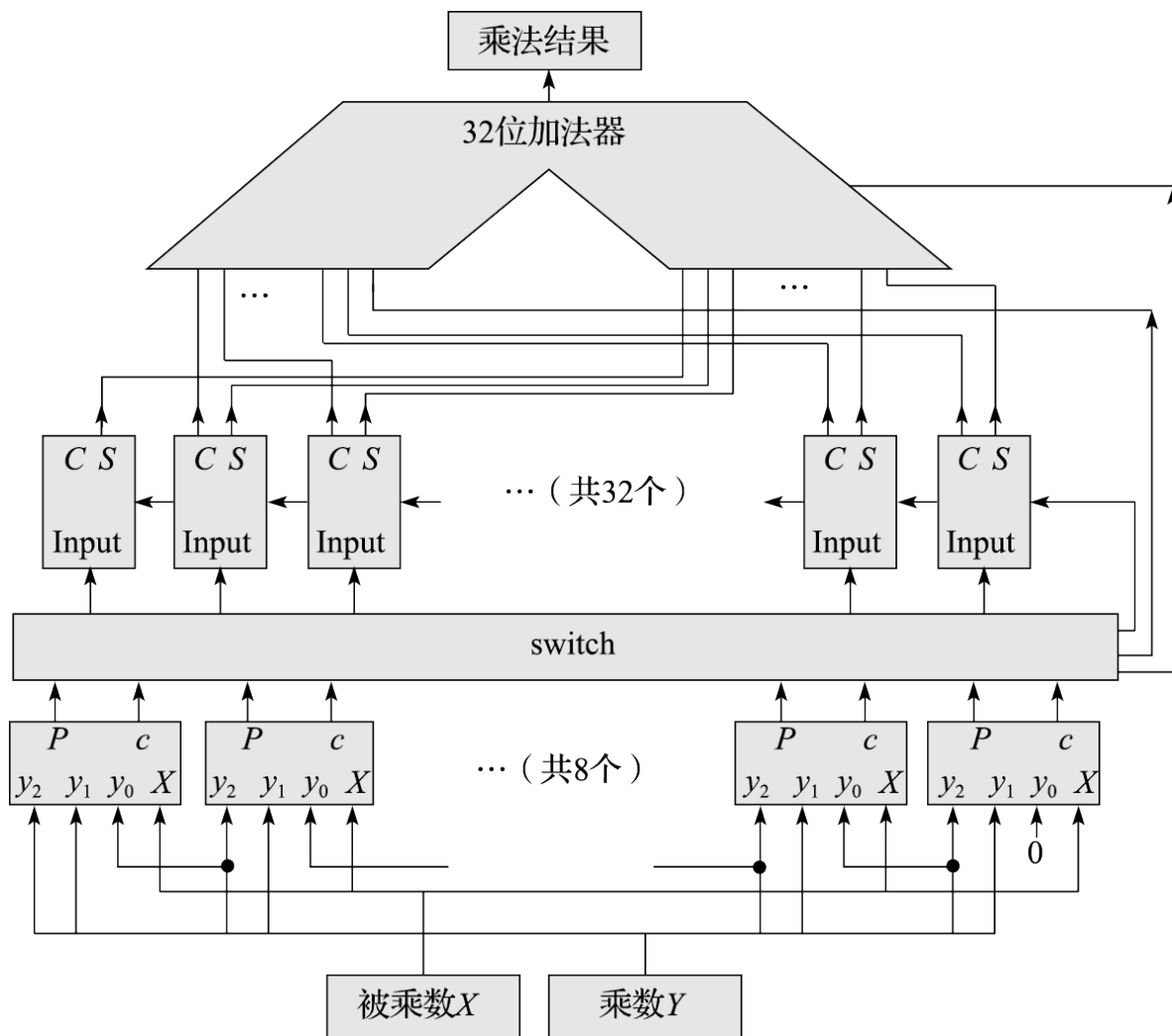
图 8.40: 16 位乘法器示意图
