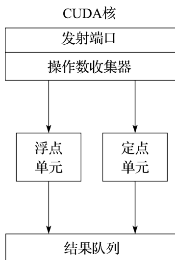
图 11.22: CUDA 核结构
