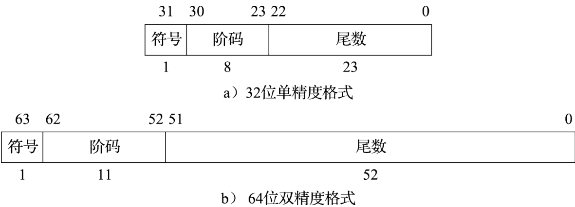
图 8.1: IEEE 754 浮点数格式
