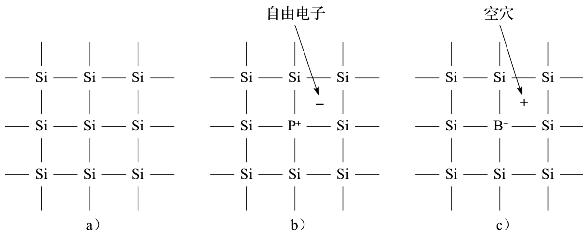
图 8.2: 半导体硅原子结构示意图
