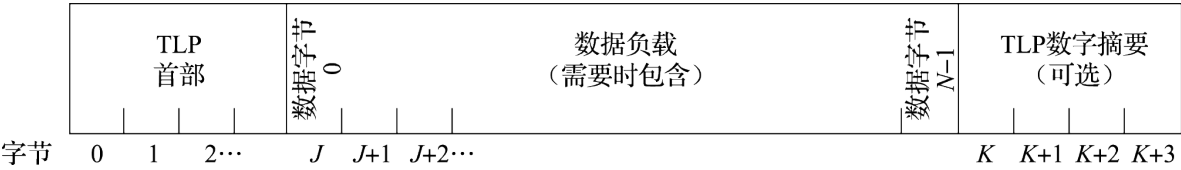
图 6.26: PCIE 总线包格式
