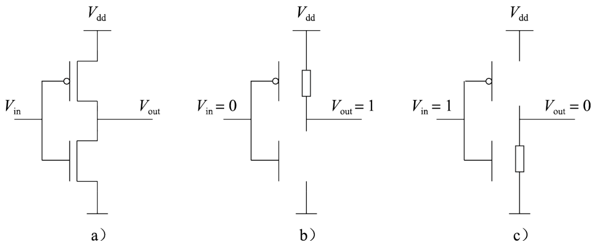
图 8.11: CMOS 电路：非门
