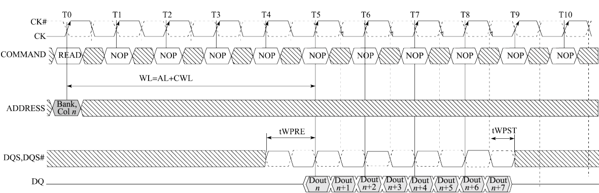
图 6.14: DDR3 SDRAM 写时序
